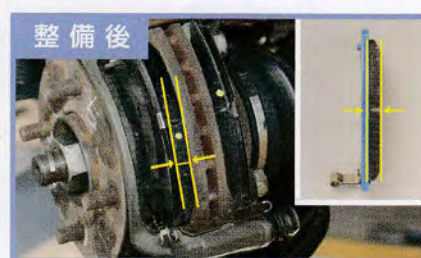
ブレーキ・パッドが新品の状態
